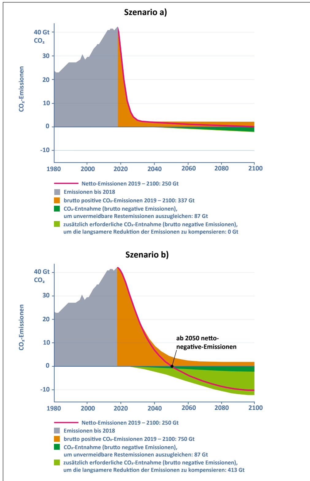
Abbildung 1: Zwei globale Szenarien zur Erreichung des 1,5°C-Ziels. In Szenario a) wird durch eine sofortige und drastische Reduktion der CO 2 -Emissionen der Bedarf an CO 2 -Entnahme auf ein Minimum reduziert. Hier müssen nur die unvermeidbaren Restemissionen ausgeglichen werden. In Szenario b) werden die CO 2 -Emissionen langsamer reduziert. Um trotzdem das 1,5°C-Ziel zu erreichen, ist in der zweiten Hälfte des Jahrhunderts CO 2 -Entnahme in sehr großem Umfang erforderlich. In der Abbildung ist nur CO 2 dargestellt, andere Treibhausgase sind nicht berücksichtigt. Quelle: Diese Grafik wurde in ähnlicher Form veröffentlicht in Fuss et al. 2020 [1] (Copyright Elsevier).
